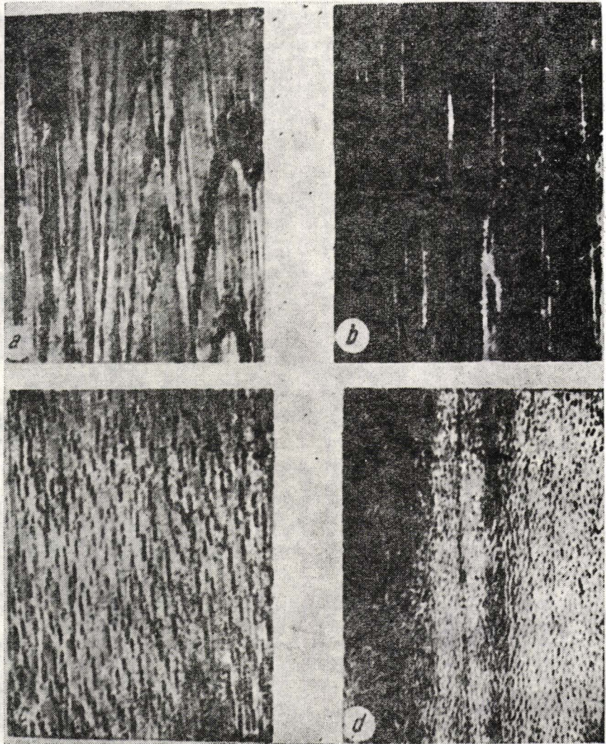
Raze medulare pe secțiune tangențială: a — la stejar; b — la cer; c — la fag; d — la platan (după Ghelmeziu și Suciu).
