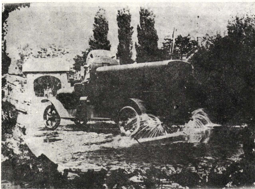
Autocisternă de 3 350 litri capacitate, fabricată în 1928 (sus), și autostropitoare produsă în 1926 pentru primăria municipiului Arad (jos)
