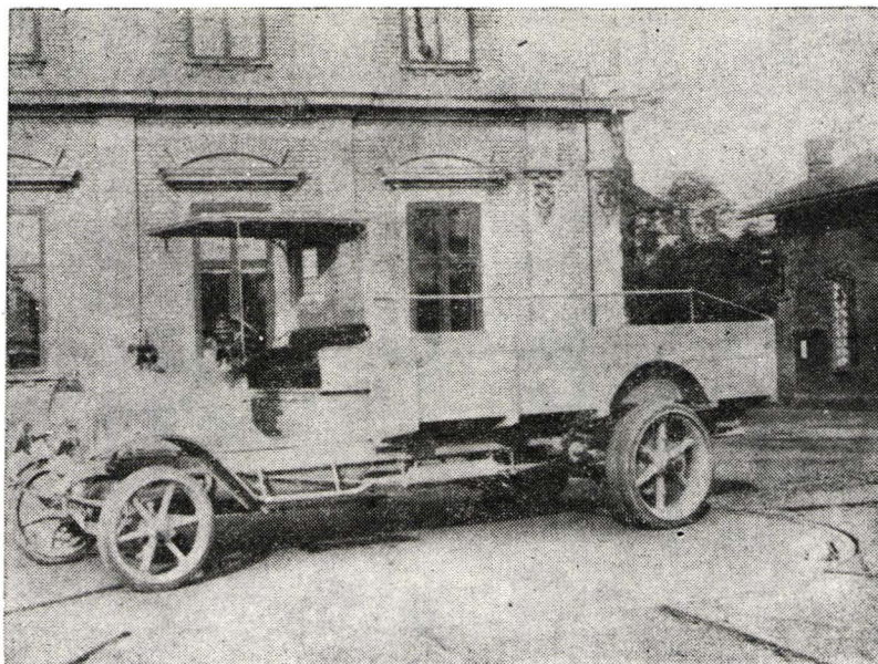
Autocamioane produse în anii 1921 (sus) și 1926 (jos) la „Astra” Arad
