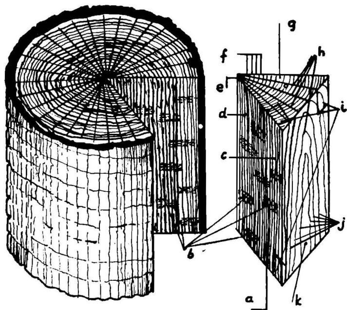
Tulpină de stejar secționată în formă de prismă triunghiulară: a — secțiune radială; b — razele medulare în secțiune radială; c — alburnul lemnului; d — inima lemnului (duramen); e — măduva; f — inelele anuale; g — secțiune transversală; h — razele medulare; i — secțiunea este mărită de 5x; j — nervură în lemn; k — secțiune tangențială. (după Iohann Flocken).
