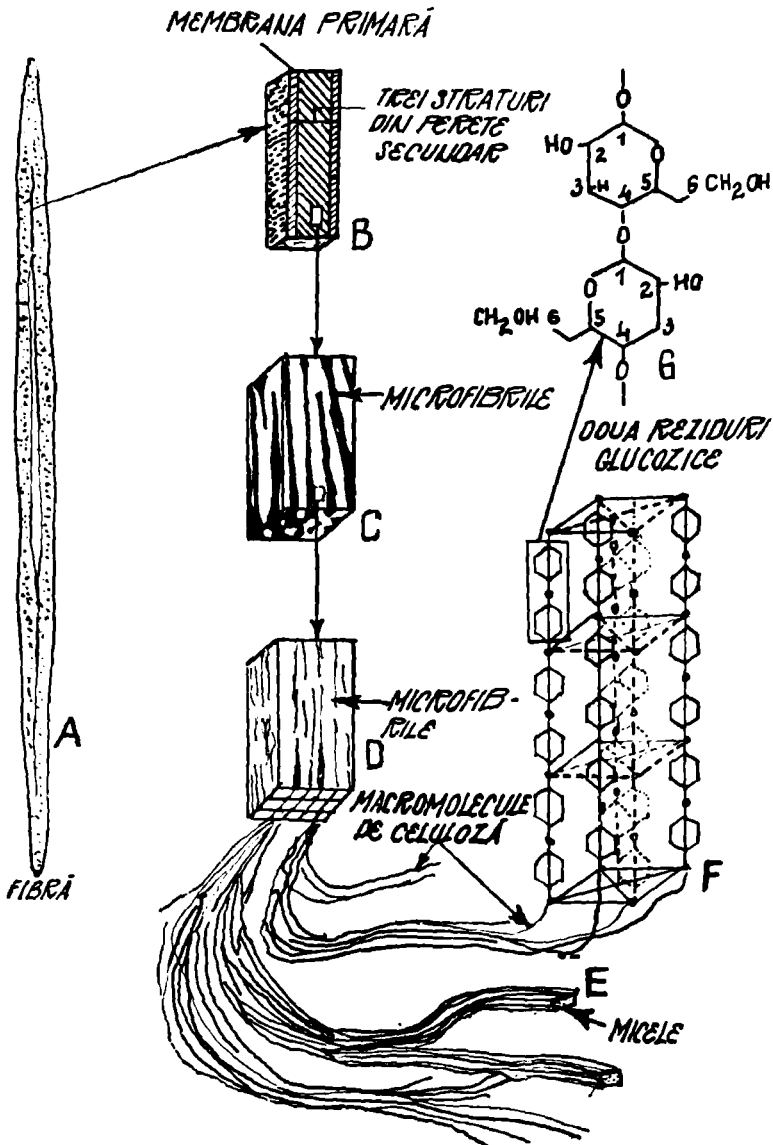
Interpretarea structurii peretelui celular (după K. Esau)
