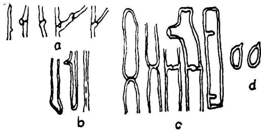
Caractere de identificare microscopică a buretelui de casă, Merulius lacrymans (după E. Vințilă); a — formarea de agrafe; b — fragmente de hife-fibre; c — hife-vase; d — spori.
