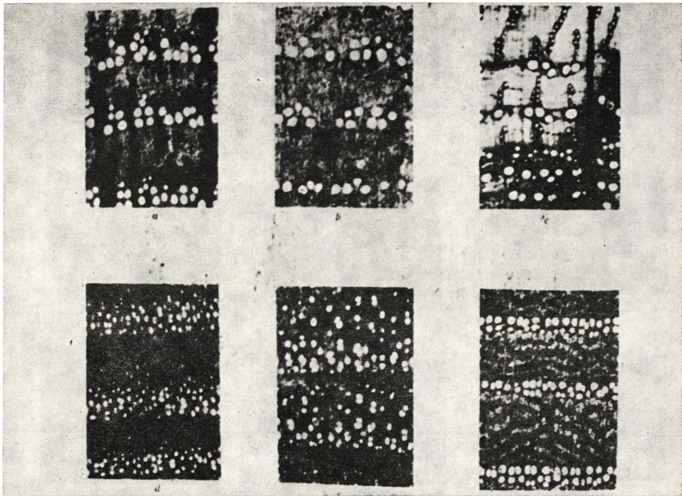
Structura macroscopică a lemnului de foioase cu porii așezați în inel (secțiuni transversale, 10\times ) (după N. Ghelmeziu și P. Suci: a — stejar; b — gorun; c — cer; d — frasin; e — salcîm; f — ulm de munte.
